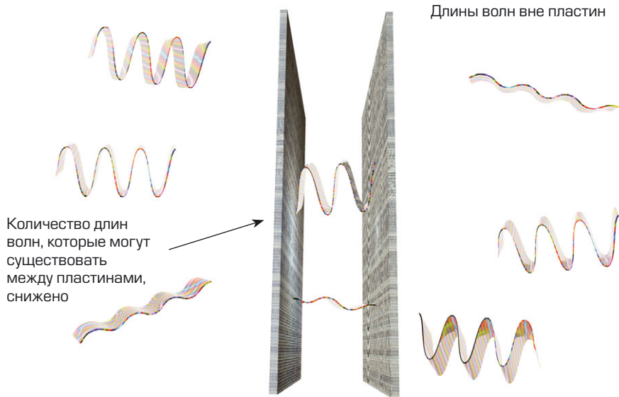
Рис. 2.11. ЭФФЕКТ КАЗИМИРА
