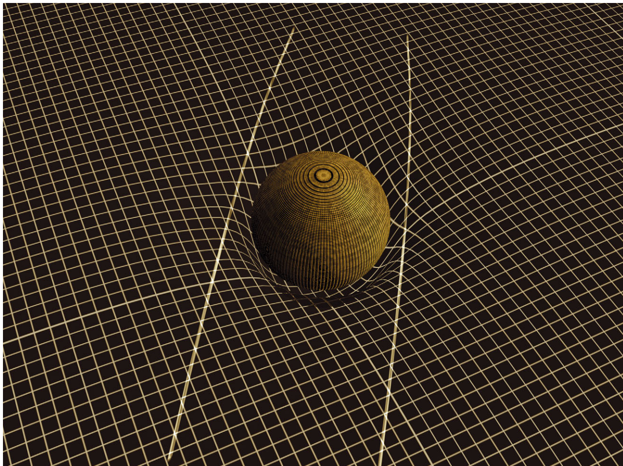
Рис. 2.7. ИСКРИВЛЕНИЕ ПРОСТРАНСТВА-ВРЕМЕНИ
