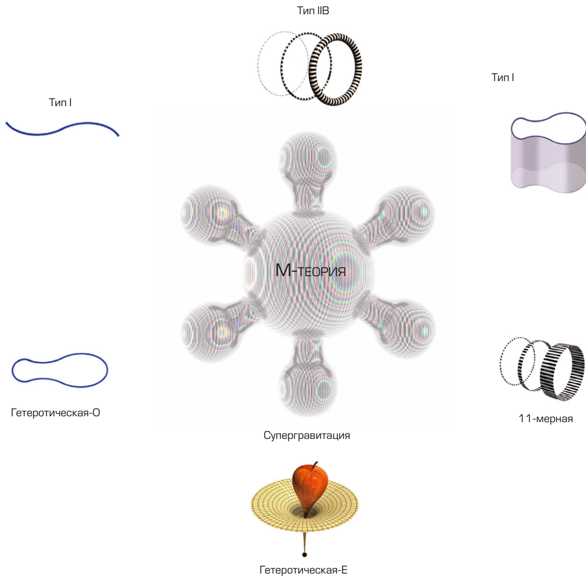
Рис. 2.16. ЕДИНАЯ ТЕОРИЯ?
