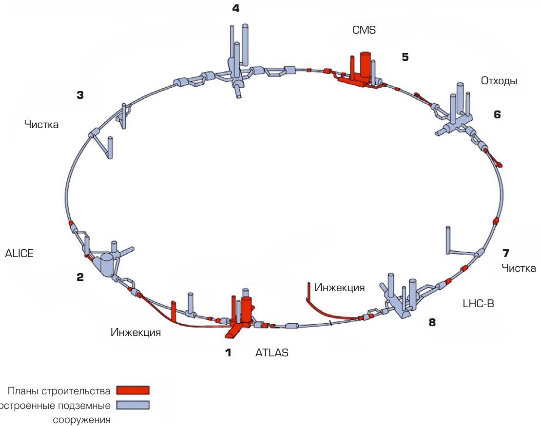
Рис. 7.20 Схема туннеля Большого электрон-позитронного коллайдера, на которой наглядно показана уже созданная инфраструктура и планы строительства Большого адронного коллайдера в Женеве.
