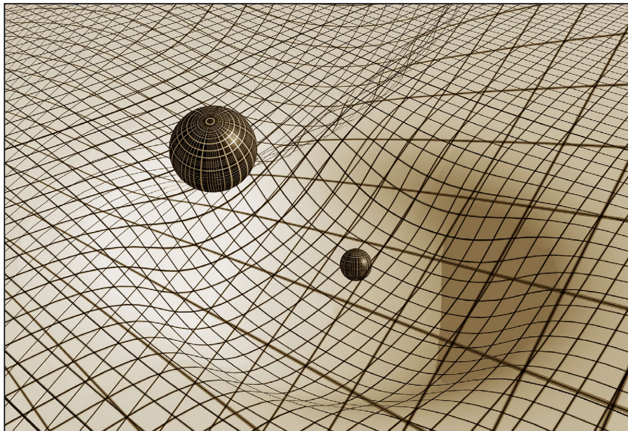
Рис. 1.12 КРИВЫЕ ПРОСТРАНСТВА-ВРЕМЕНИ
