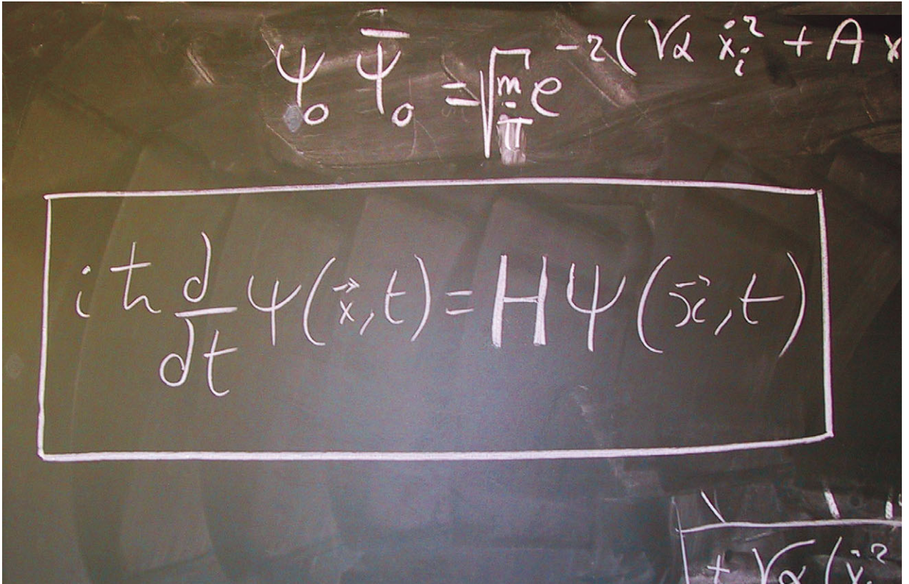
Рис. 4.5 УРАВНЕНИЕ ШРЁДИНГЕРА
